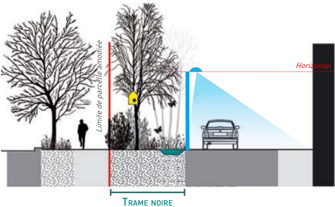
Schéma d'orientation de projecteurs sur façade :
